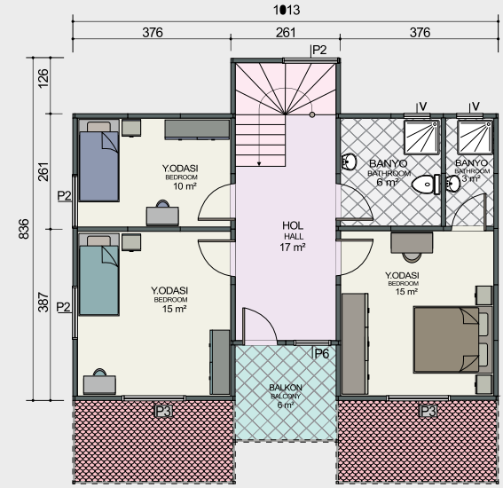
1. Kat Planı / First Floor Plan 66 m 2 + 6 m 2 = 72 m 2
